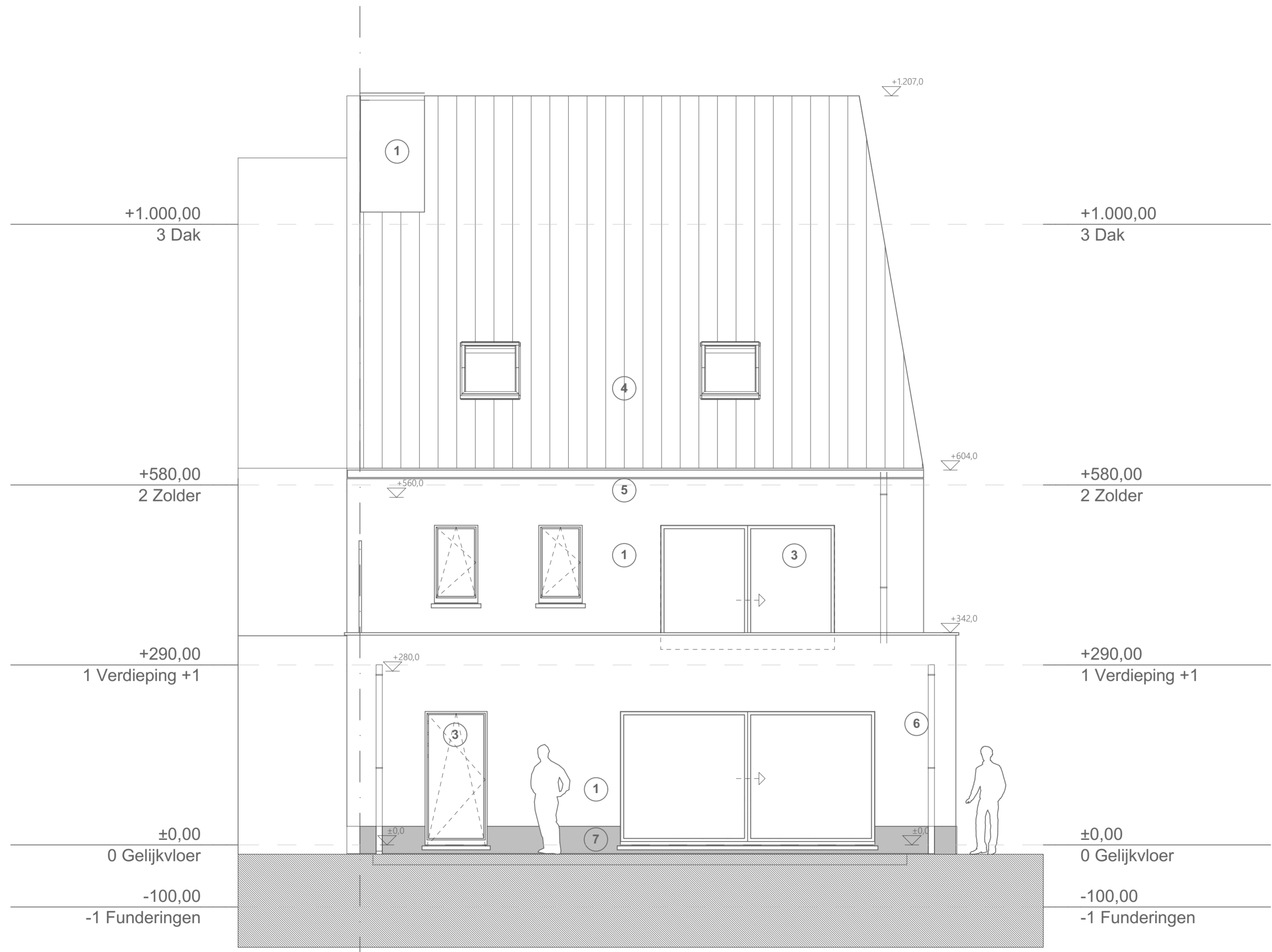
ACHTERGEVEL NIEUWE TOESTAND
