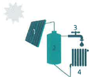
1. Zonnecollector | 2. Opslagvat zonneboiler | 3. Sanitair warm water | 4. Afgifte-element voor ruimteverwarming (oplozeel)
